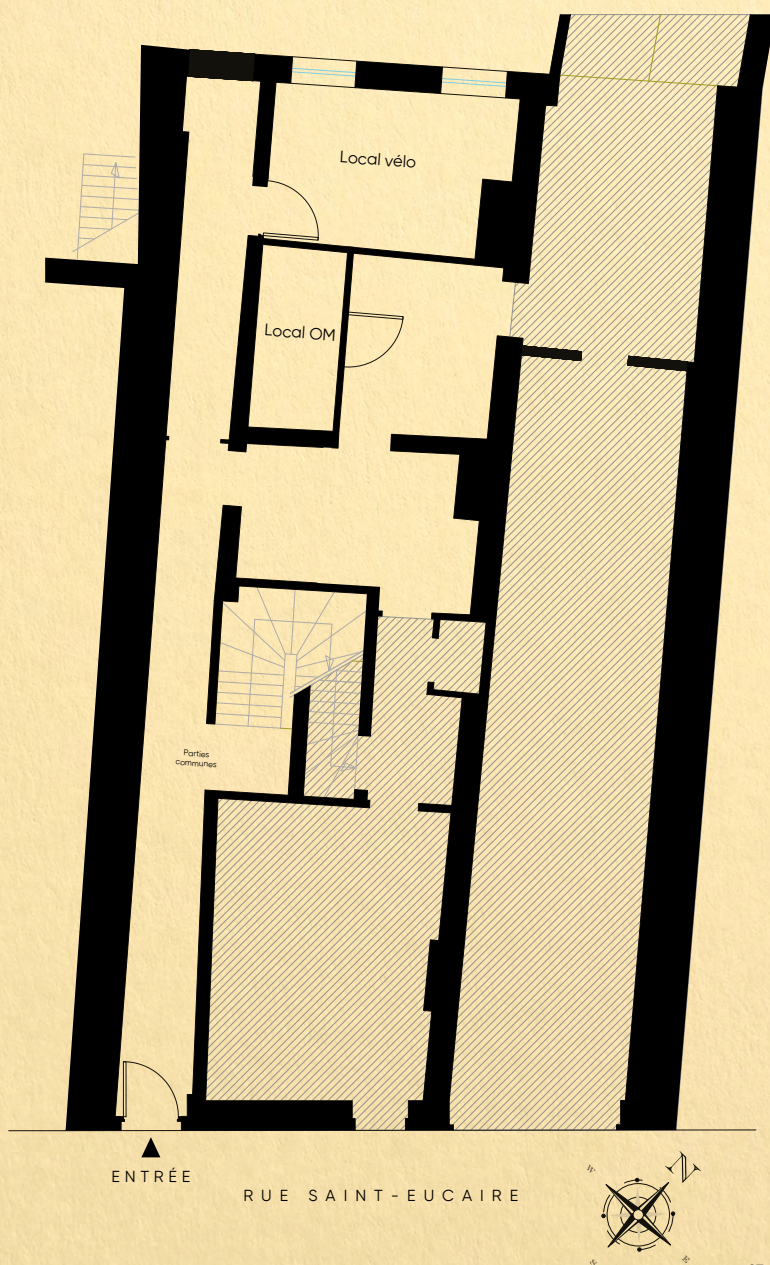
Rez-de-chaussée
